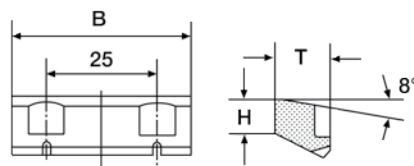
Ausführung: C ab B= 38 mm
